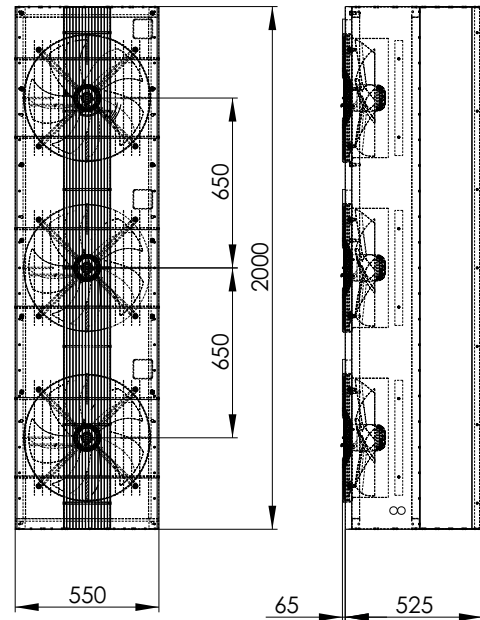
Fig. 5 VCP-03-200 module - air-only Рис. 5 Модуль VCP-03-200 - холодный
